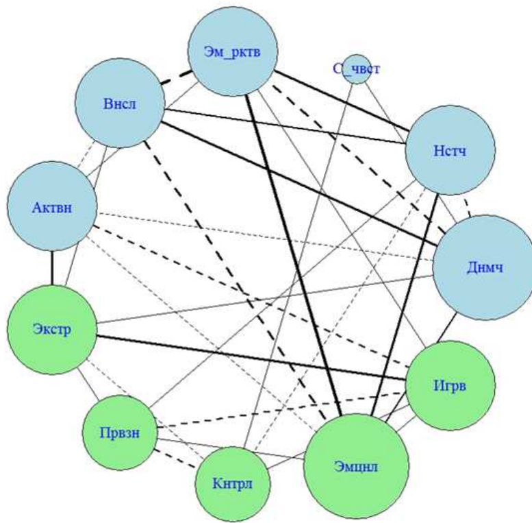
Рис. 3. Корреляционный граф
