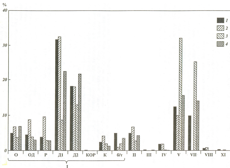
Рис. 2. Типоморфные особенности алмазов из современных россыпей Анабарского алмазного района.
