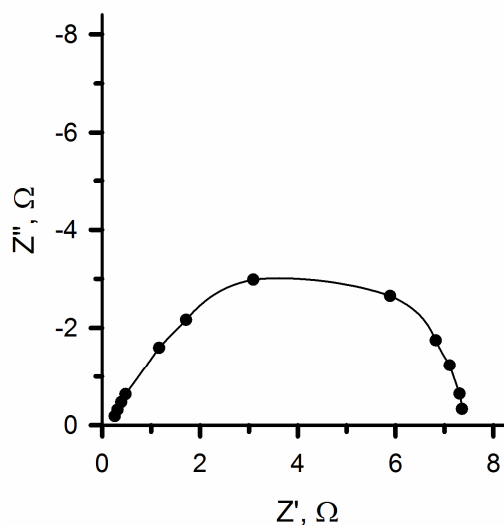
Рис. 9. Нодограф импеданса для конденсатора С9
