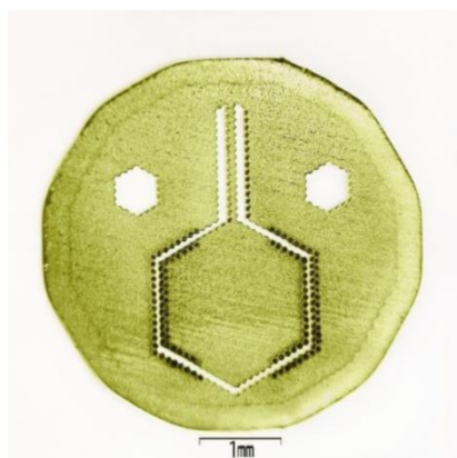
Рис. 1. Прототип стеклянного ММА
