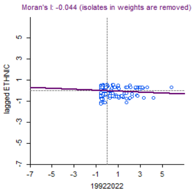
Рис. 5. Индекс пространственной автокорреляции Морана, рассчитанный для стран
