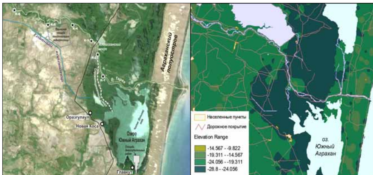
Рис. 2. Карта-схема реализации рассматриваемых вариантов обеспечения терской водой залива Южный Аграхан
