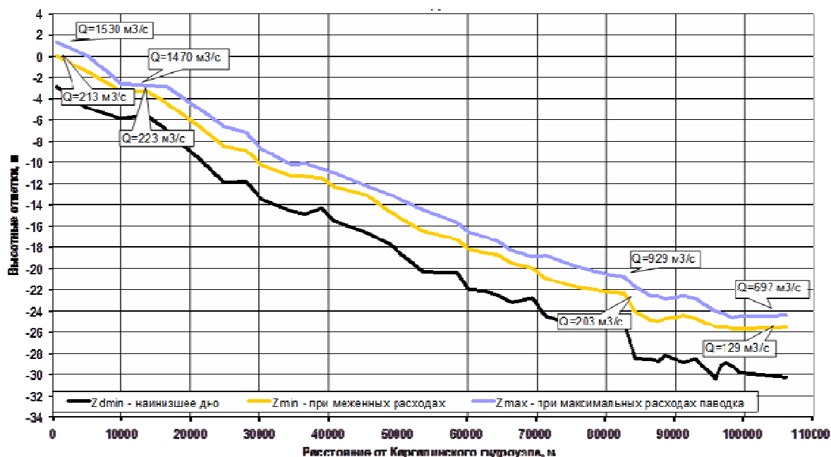
Рис. 4. Результаты численного моделирования гидродинамических процессов на устьевом участке р. Терк при паводках различной обеспеченности с помощью гидравлического модуля Streamflow1
